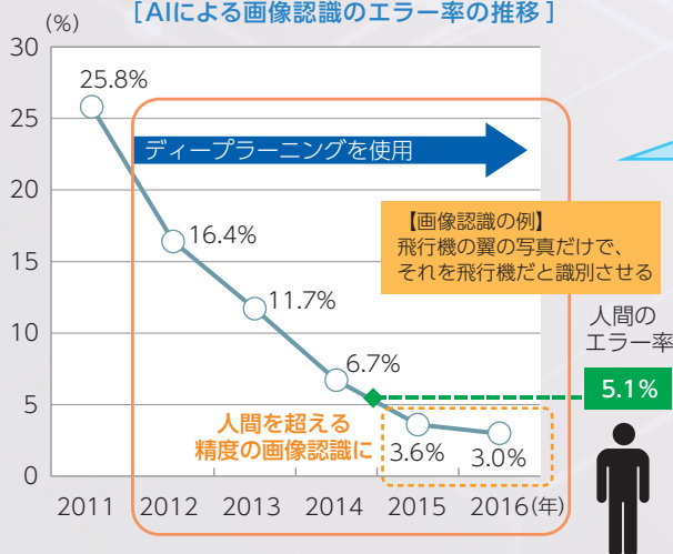
【AIによる画像認識のエラー率の推移】
